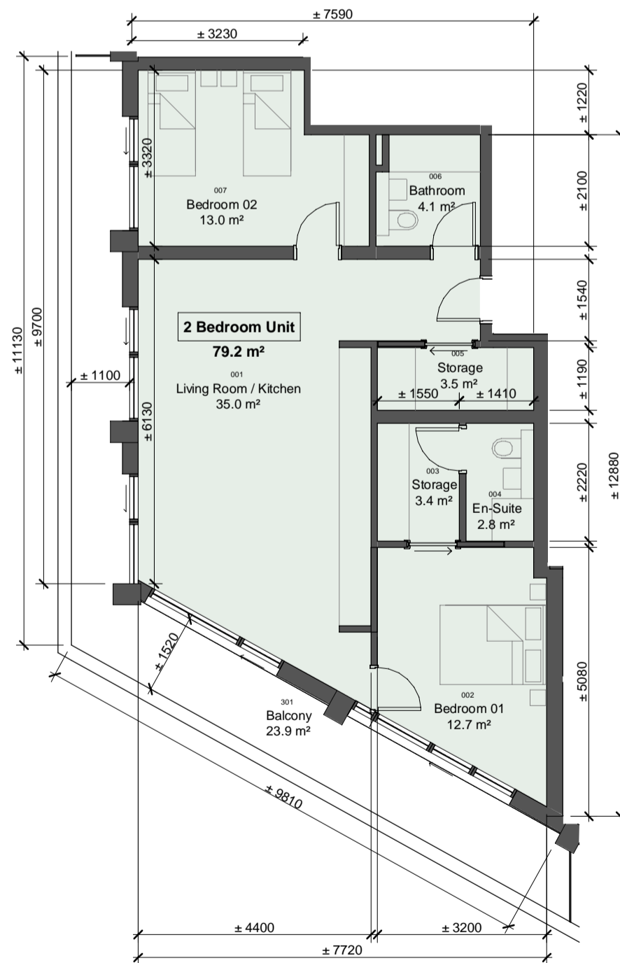
4 Unit Type 2BR-J-2 scale 1 : 100
