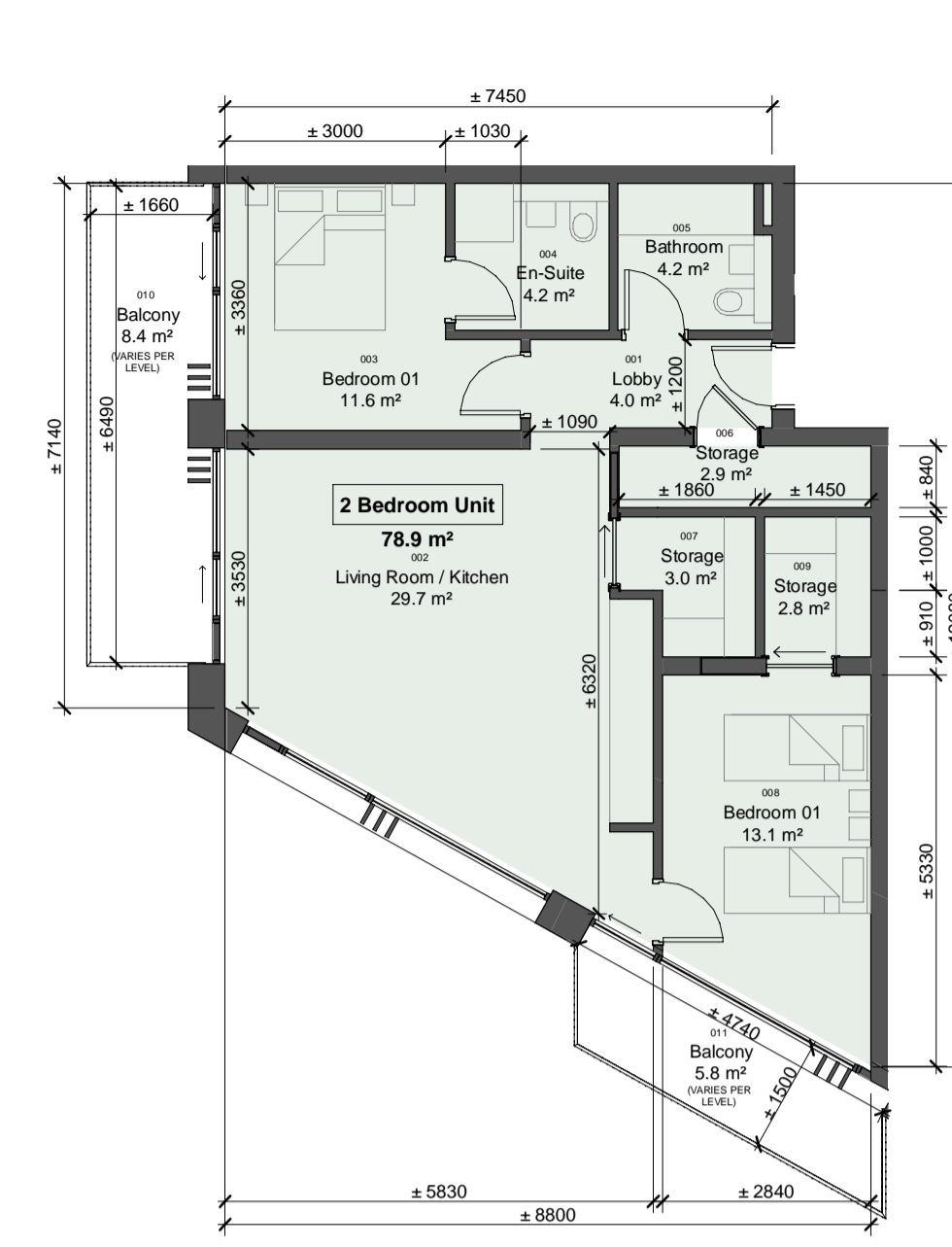
3 Unit Type 2BR-J-1 scale 1 : 100
